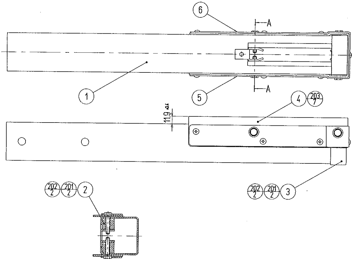
SECTION A-A
